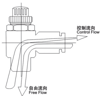
SL排气控制(标准型) SL Exhaust Control(Standard Type)
